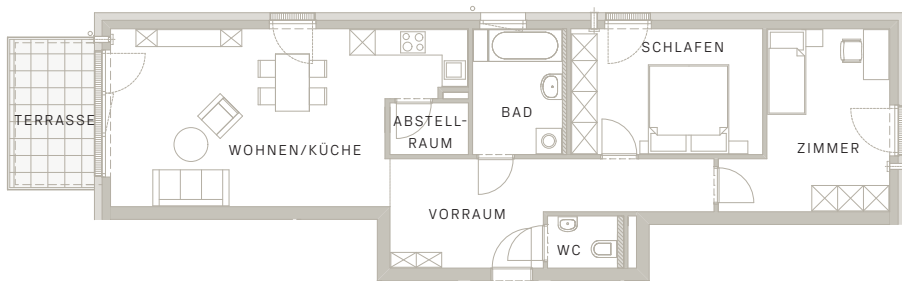
ERDGESCHOSS HAUS 24A
